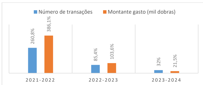
Gráfico 7 - Evolução de Operações nos POS's
