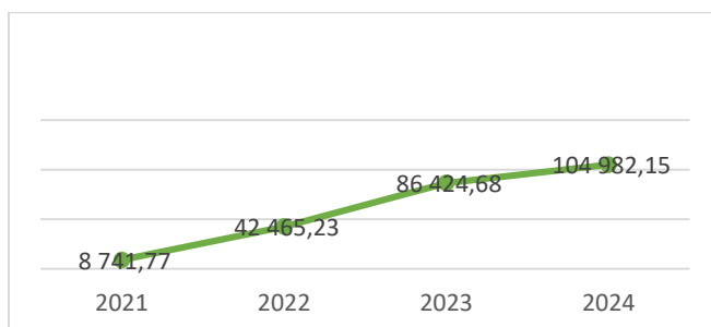
Gráfico 6 - Montante Gasto em POS's (mil dobras)
