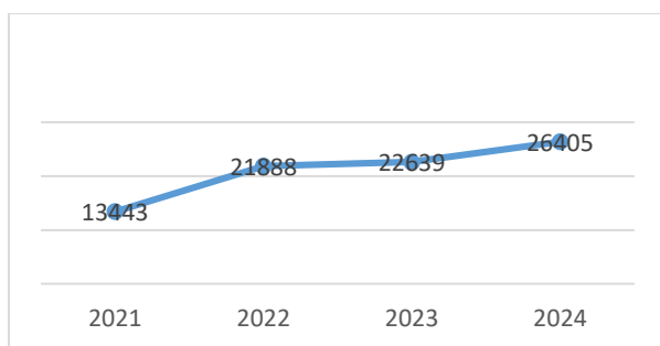
Gráfico 1 - Nº de Levantamentos em ATM
