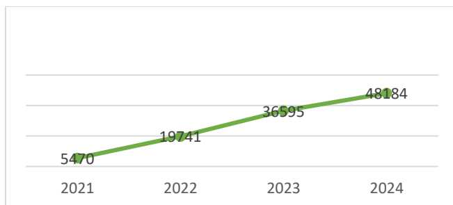
Gráfico 5 - Nº de Compras em POS
