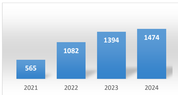
Gráfico 4 - Nº de Consultas por ano em ATM
