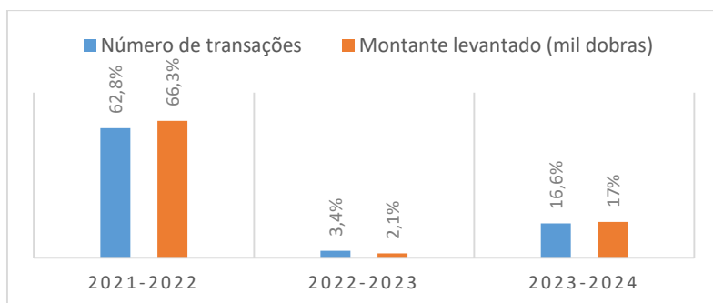
Gráfico 3 – Evolução de operações nos ATM's
