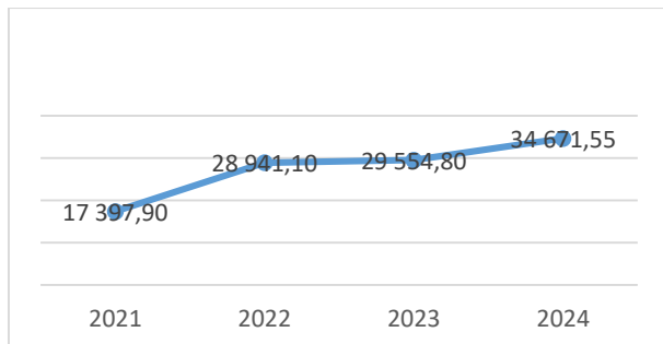
Gráfico 2 - Montante Levantado nos ATM's (mil dobras)
